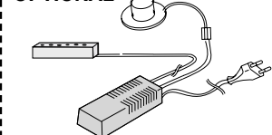
IMPIANTO TRASFORMATORE 10W-12V DC PER EASY-LED 1 TRASFORMATORE X 6 LUCI 1 TRANSFORMER ON 6 LIGHTS 1 ТРАНСФОРМАТОР НА 6 ЛАМП W. 5 D. 4 H. 4 Vol. 0,03 kg 1 CO 000VT1.01AL01 € 40
